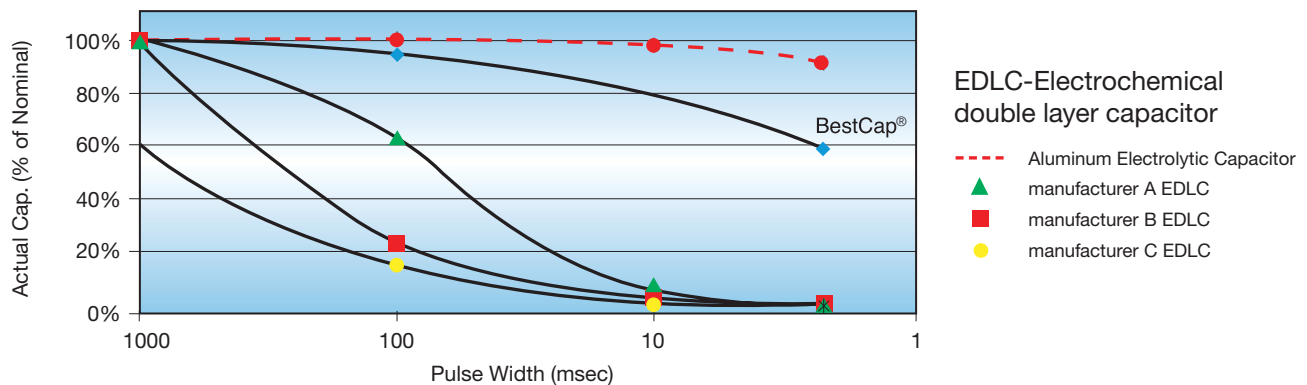
Figure 2. Actual Capacitance vs. Pulse Width
